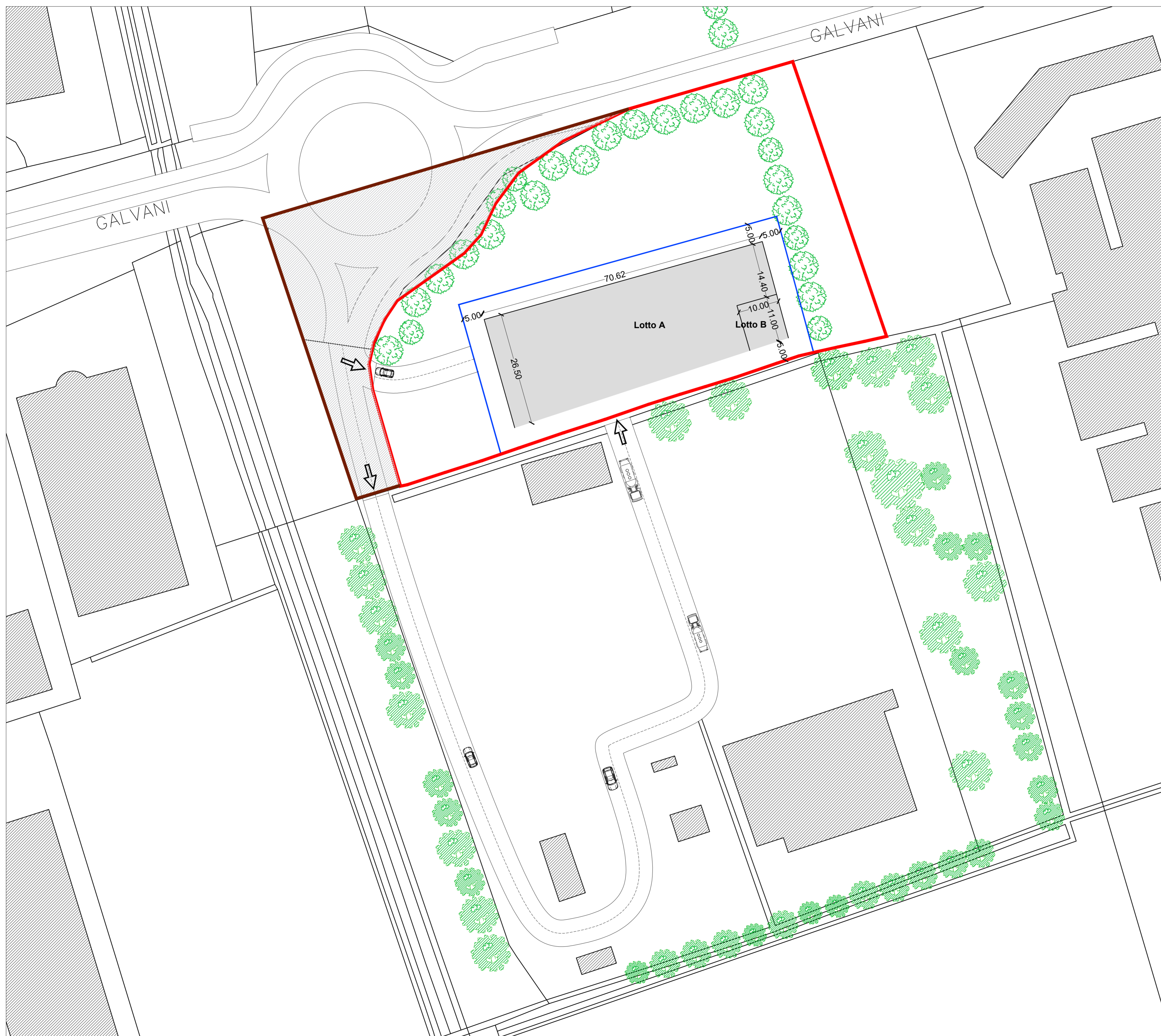
PLANIMETRIA GENERALE IN PROGETTO SC. 1:500
