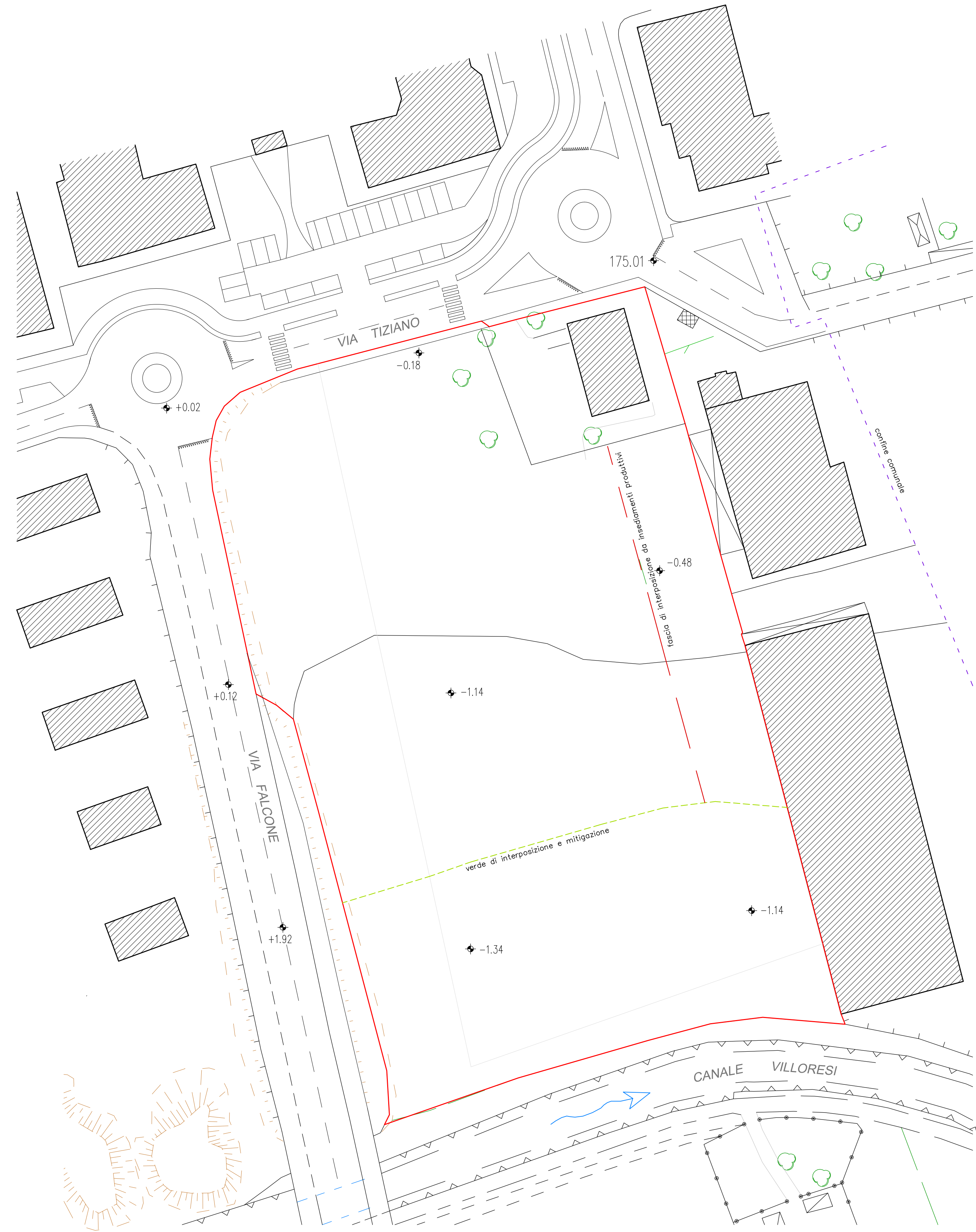
PLANIMETRIA STATO ESISTENTE - SCALA 1:500
